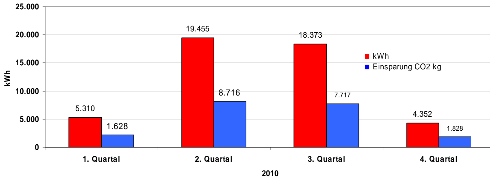
PV Anlage Otto-Hahn-Schule 50,4 kWpeak: Einsparung in kg
