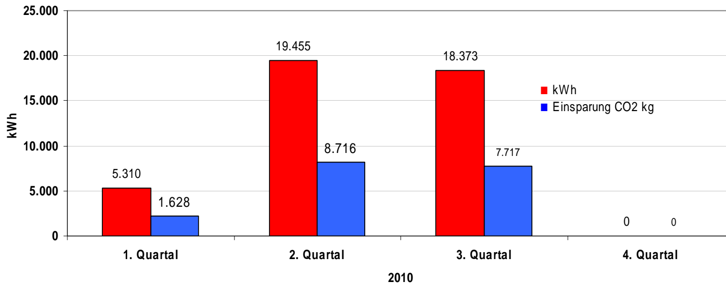
PV Anlage Otto-Hahn-Schule 50,4 kWpeak: Einsparung in kg
