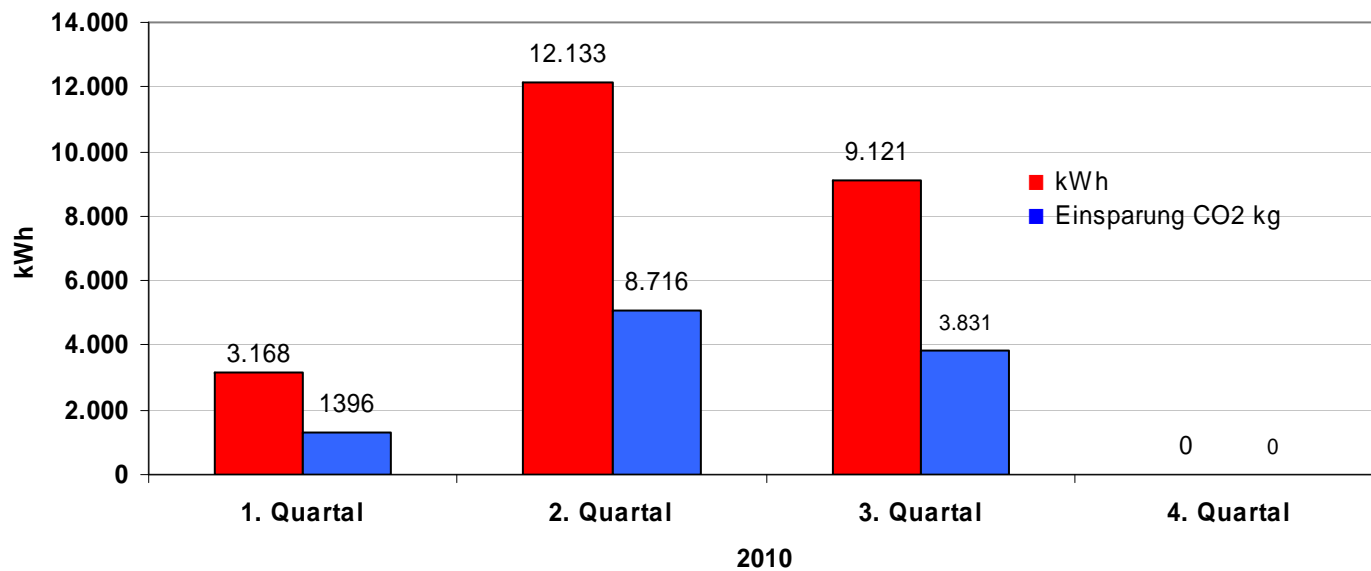
PV Anlage Erich Kästner Schule 25,16 kWpeak: Ertrag in kWh/CO 2 Einsparung in kg
