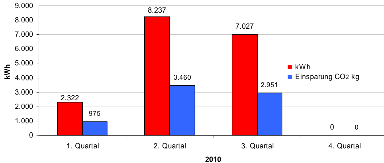
PV Anlage Eichendorfschule 21,84 kW peak : Ertrag kWh/Einsparung CO 2 in kg
