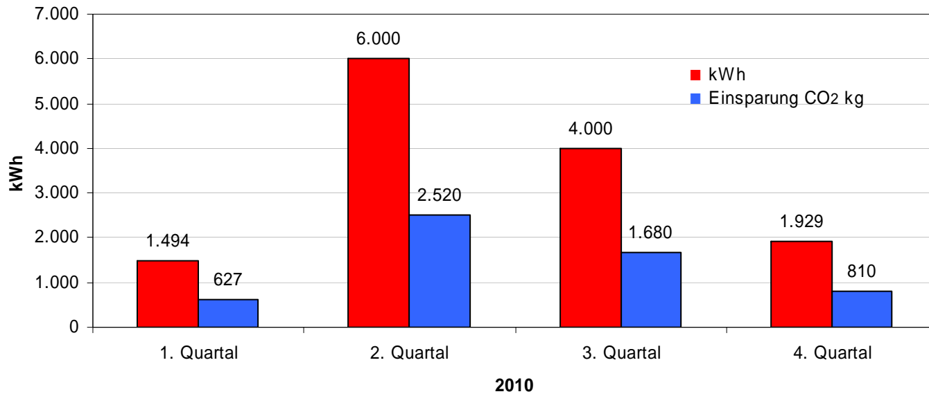
PV Anlage Anne-Frank-Schule 22,12 kW peak : Ertrag kWh/CO 2 Einsparung in kg
